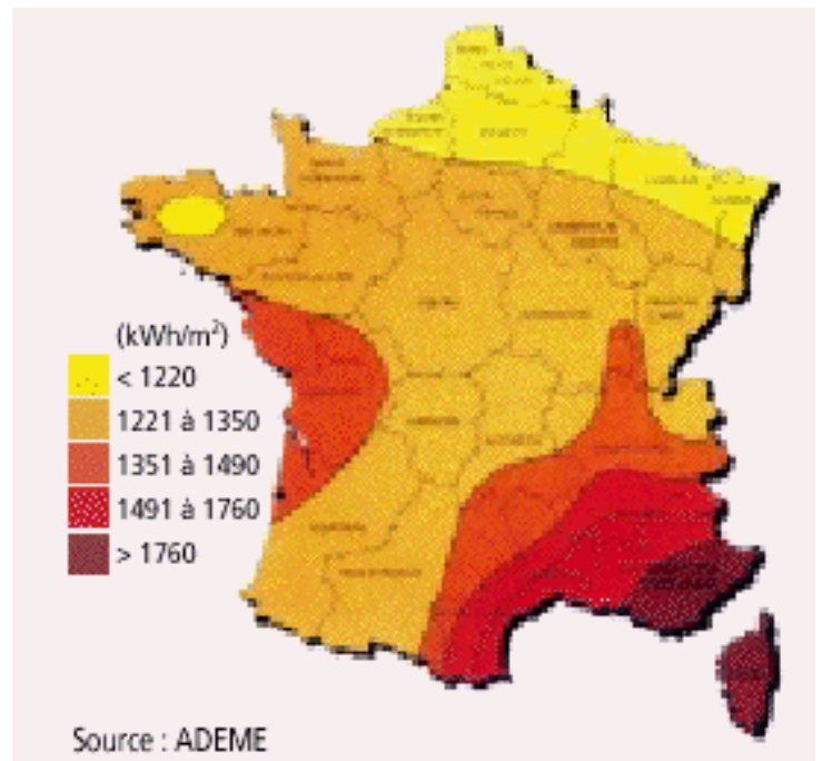
Gisement solaire en kWh/m 2 et par an
