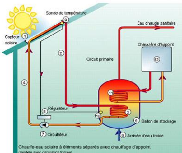
Energie solaire thermique : chauffage domestique
