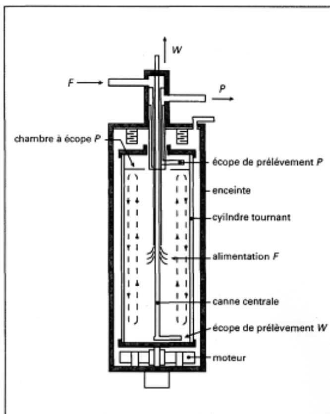
Figure 1 Schéma d'une centrifugeuse. L'alimentation du gaz (F) est assurée par la canne centrale. L'écope de prélèvement W permet de récupérer la fraction de gaz appauvrie en éléments légers, notée W, alors qu'une seconde écope garantit l'extraction de la fraction enrichie, notée P
