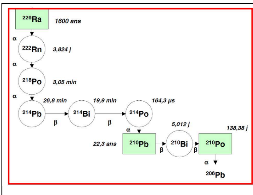
Figure 1 : Chaîne de désintégration du Ra 226 ►
