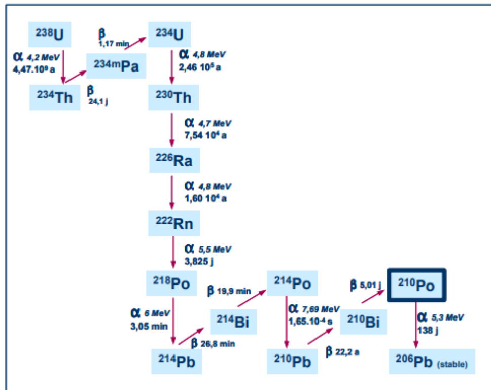
Figure 1 : Chaîne de décroissance radioactive du Polonium
