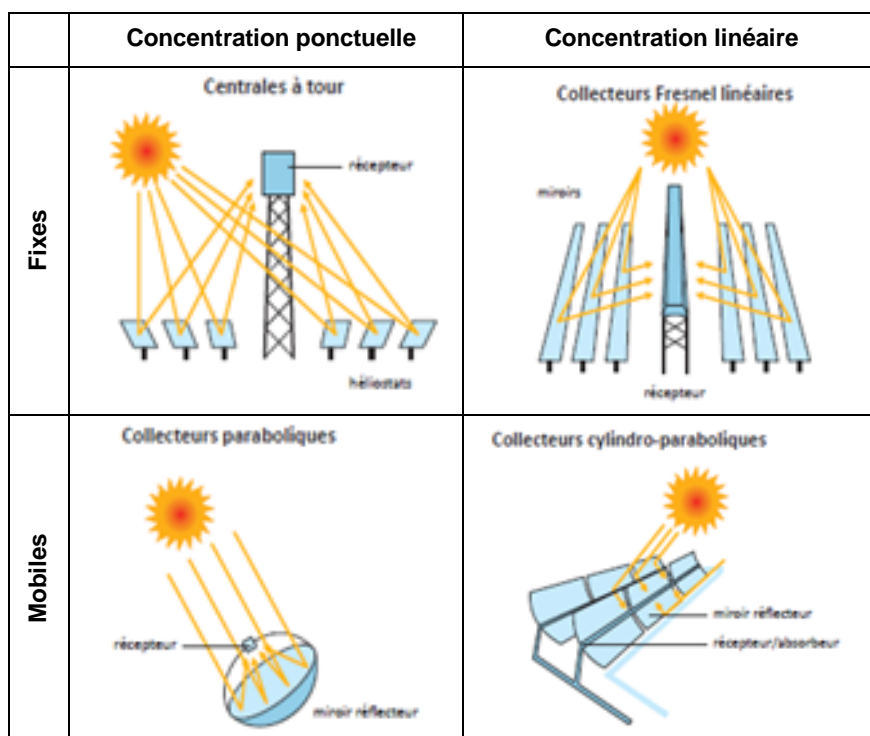
Figure 1 : Centrales à capteurs cylindro-paraboliques
