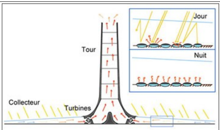
Figure 2 : Principe d'une centrale à effet de cheminée
