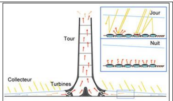
Figure 2 : Principe d'une centrale à effet de cheminée
