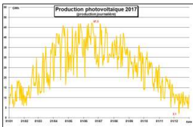
Figure 8 : Production photovoltaïque annuelle (mesures journalières)
