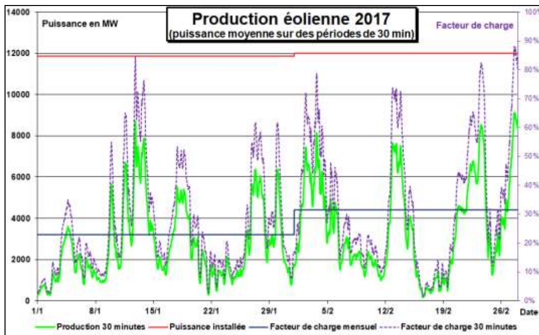
Figure 6 Production éolienne mensuelle et facteur de charge (source RTE)
