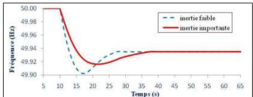
Figure 3 : Effet amortisseur de l'inertie sur la réponse du réseau en fréquence (Source EDF R&D)
