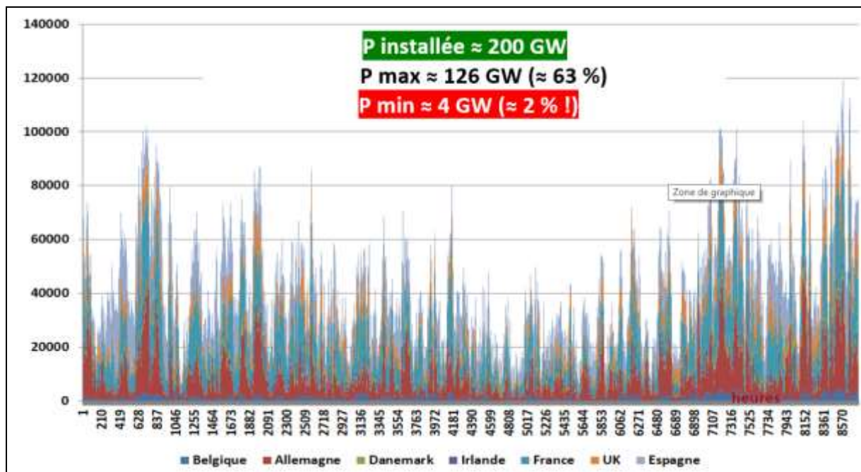
Figure 7 : Production éolienne cumulée au pas horaire de 7 pays européens en 2025-2030, pour un climat identique à celui de 2013 (Source Techniques de l'Ingénieur)
