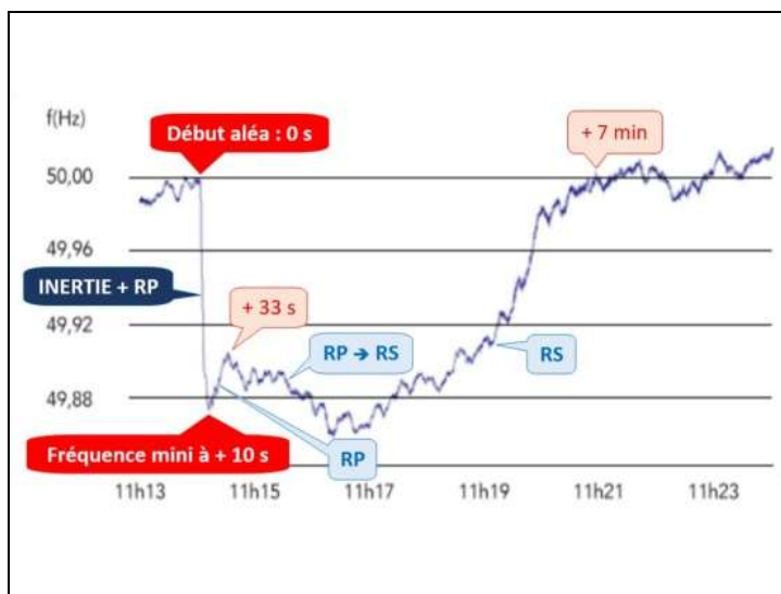
Figure 5 : Exemple réel de perturbation due à perte de production de 2 800 MW
