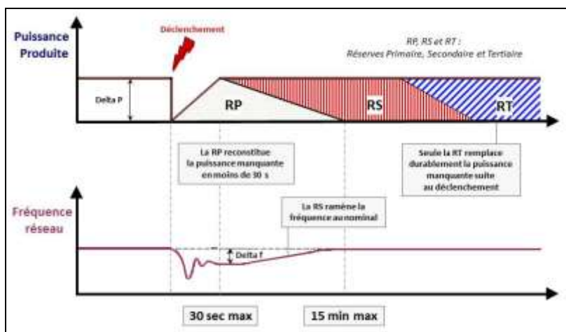
Figure 4 : Réactions des réserves primaires, secondaires et tertiaires suite à un incident sur le réseau
